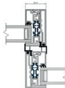
Slim Interlock
